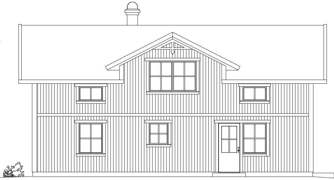
FASAD FRÅN SÖDER
